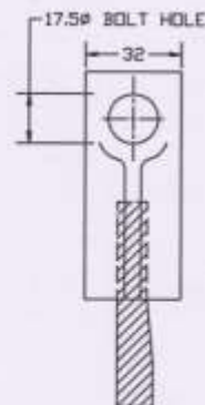
DETAIL OF LUG
